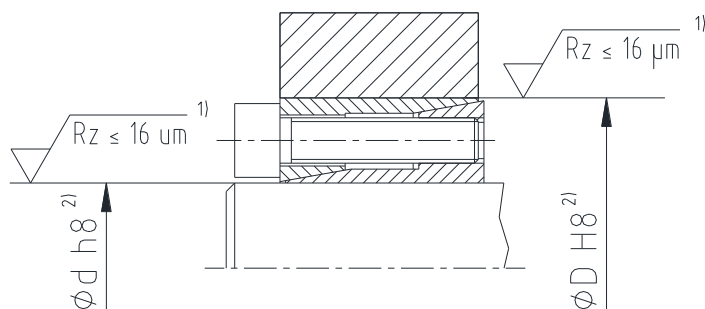
rysunek 3: tolerancje i chropowatość powierzchni (przykład: CLAMPEX® KTR 105)
