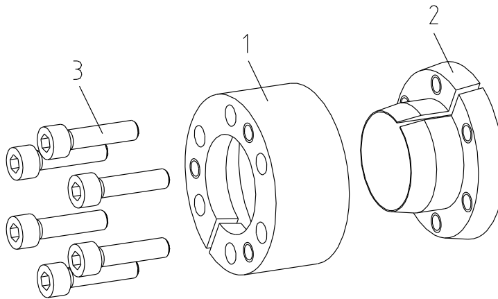
rysunek 2: CLAMPEX® KTR 105
