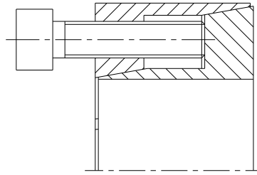
rysunek 4: montaż pierścienia rozprężno-zaciskowego
