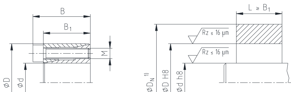
rysunek 1: wymiary - CLAMPEX® KTR 105
