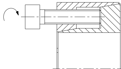
rysunek 5: zluźnianie pierścienia KTR 105
