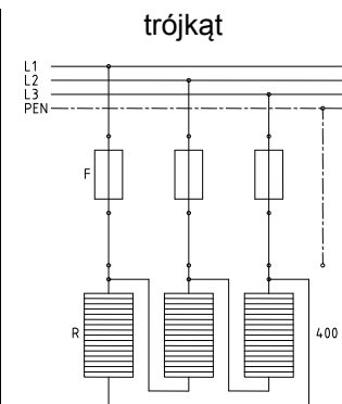
rysunek 14: schemat połączeń bez termostatu – 400 V
