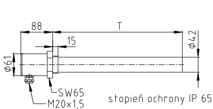
rysunek 1: typ EHP – G 1 1/2" bez regulacji temperatury
