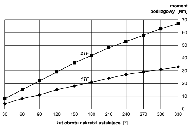
diagram 2: RUFLEX® rozmiar 01
