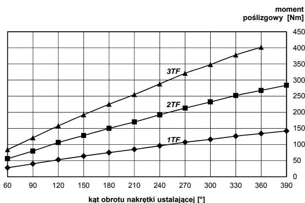
diagram 4: RUFLEX® rozmiar 2
